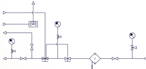
Схемы газопроводов
